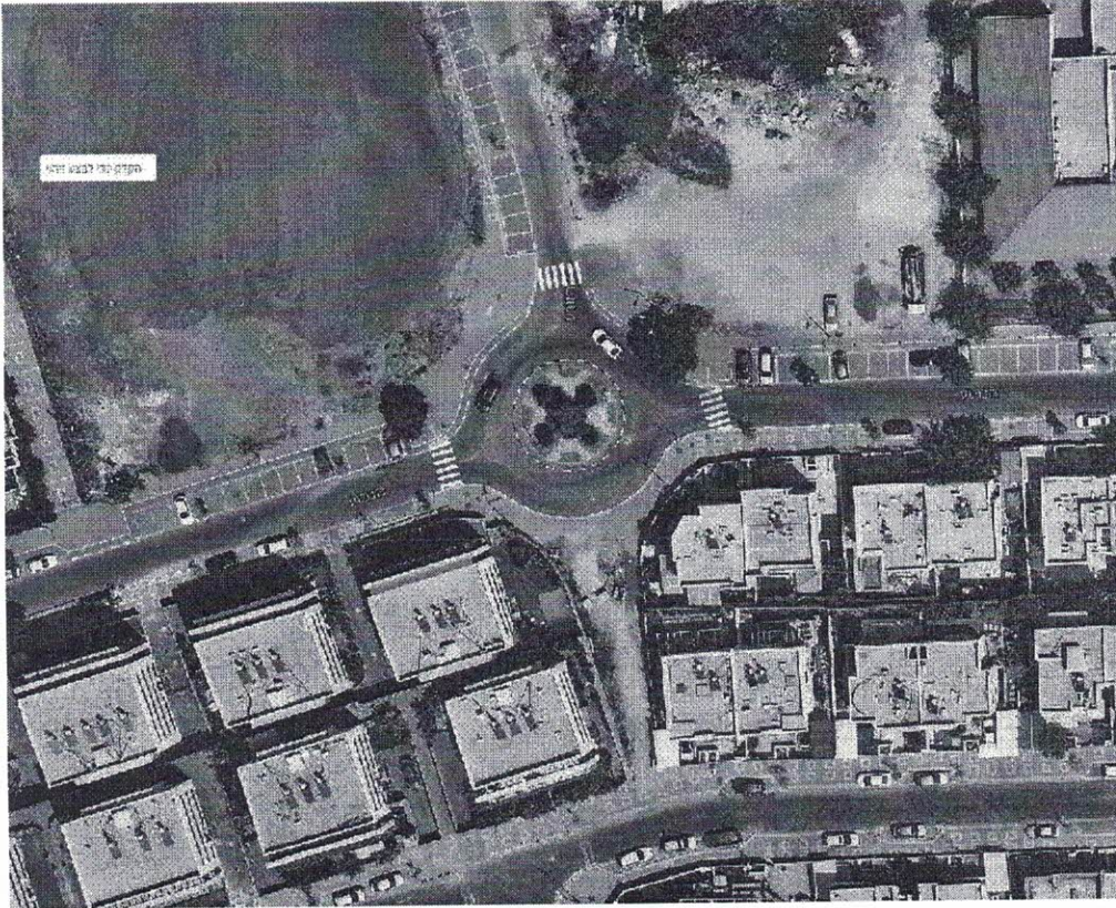
תרשים 3: מעברי הציה במעגל תנועה הנוטע/הזורע.
