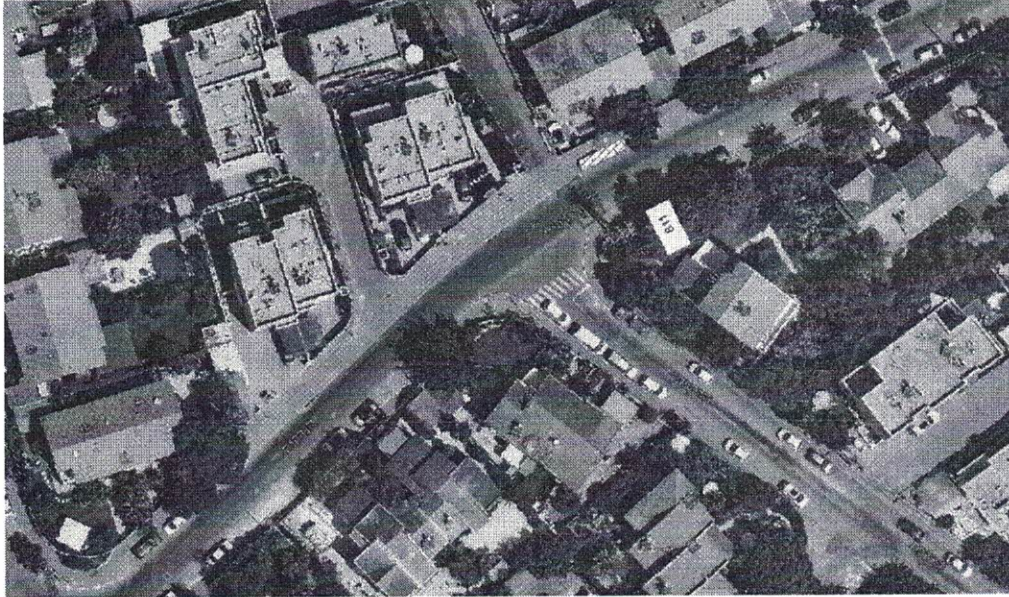
תרשים 5: מעבר חציה ברחוב הנרקיס פינת רחובה הרקפת
