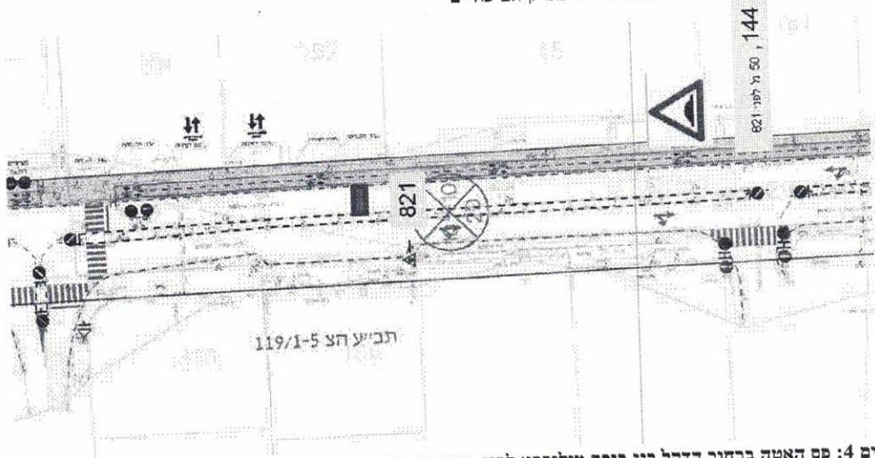
תרשים 4: פס האטה ברחוב הדקל בין כיכר מוליבבא לבין רחוב היסמין
